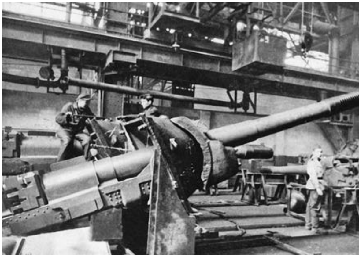
Сборка САУ ИСУ-152: гаубица-пушка МЛ-20С
