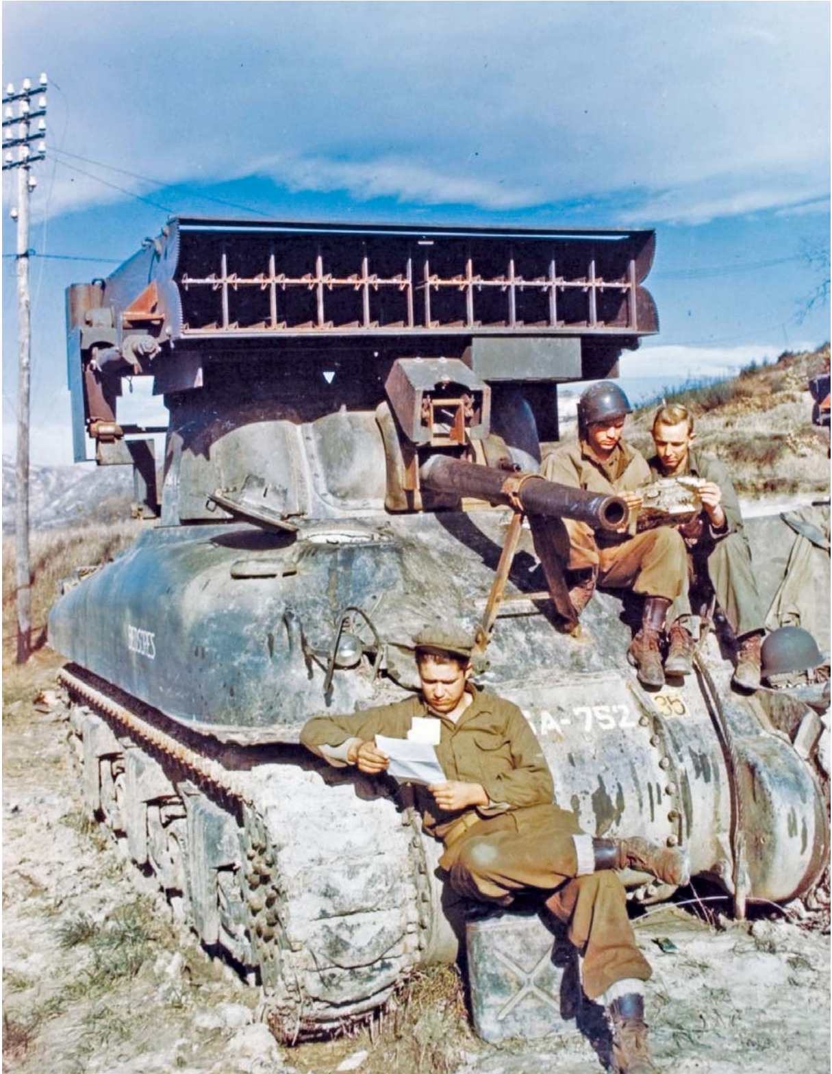
Танк «Шерман» с системой залпового огня
