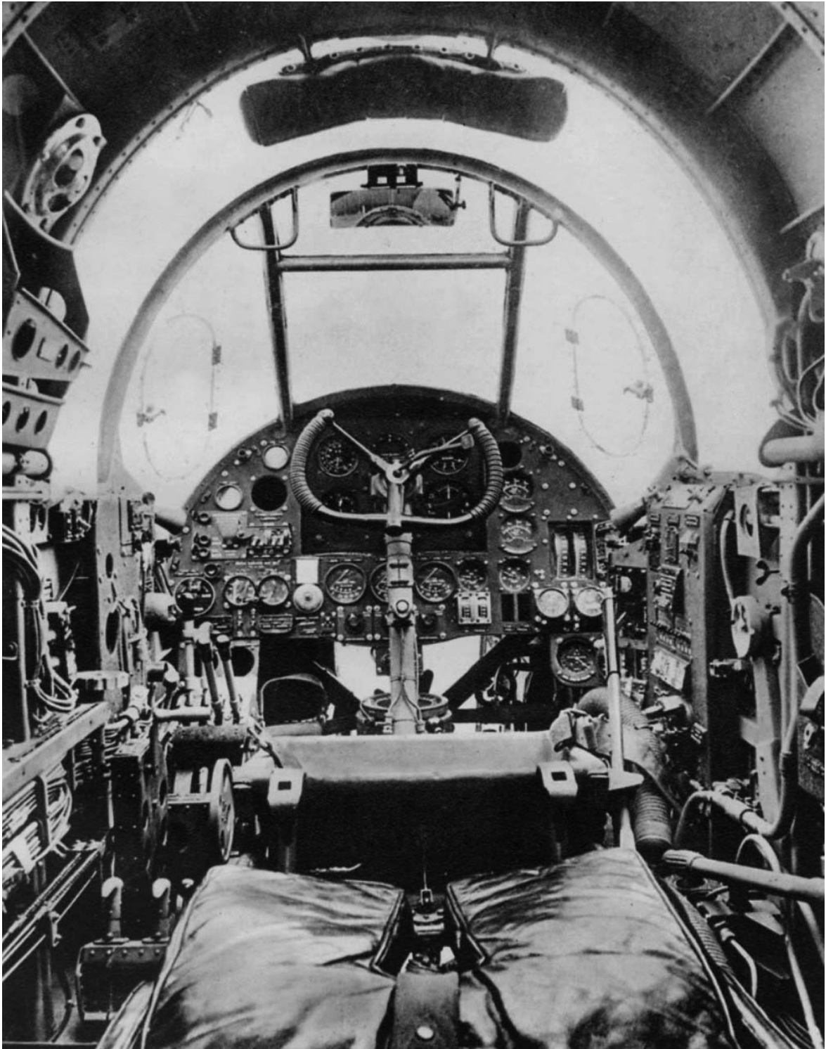
Кабина пилота английского бомбардировщика
