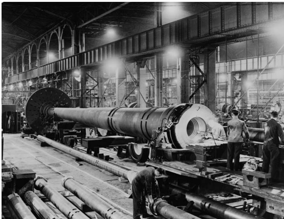
Цех английского завода по производству 406-мм морских орудий
