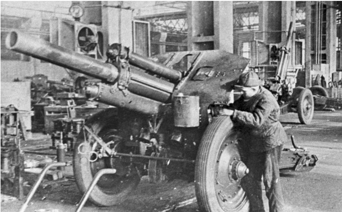
Сборка 122-мм гаубиц М-30
