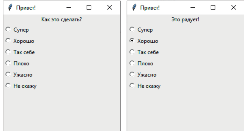
Рис. 8.3. Результат работы версии программы с переключателем
