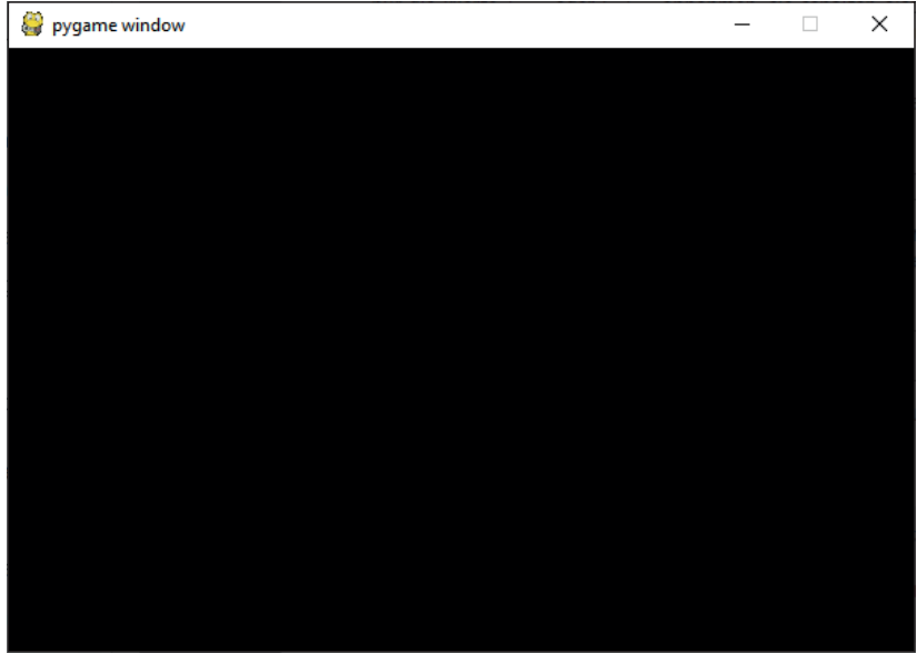
Рис. 13.1. Окно pygame
