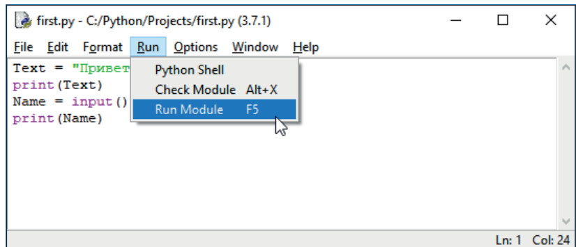
Рис. 1.18. Запуск программы
