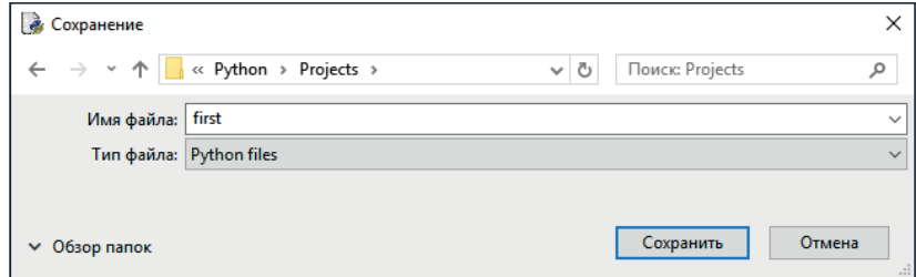
Рис. 1.17. Сохранение файла
