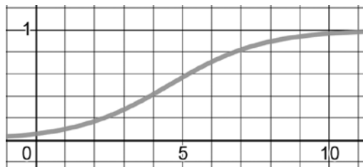
Рис. 6.6. График логистической функции
