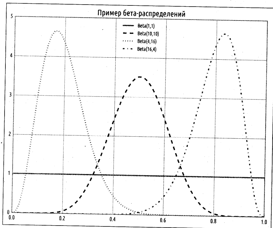
Рис. 7.1. Пример бета-распределений
