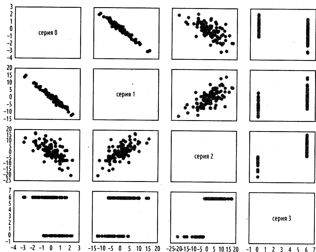
Рис. 10.4. Точечная матрица
