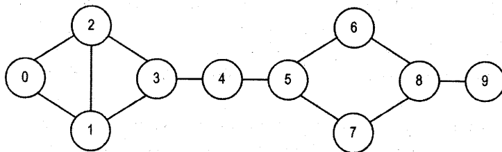
Рис. 1.1. Сеть DataSciencester
