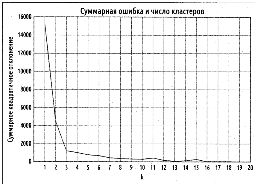
Рис. 19.4. Выбор k
